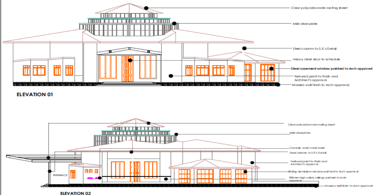
ELEVATION 02
